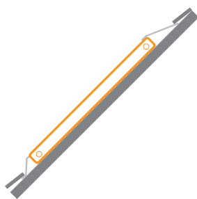
Montage intégré dans la toiture
