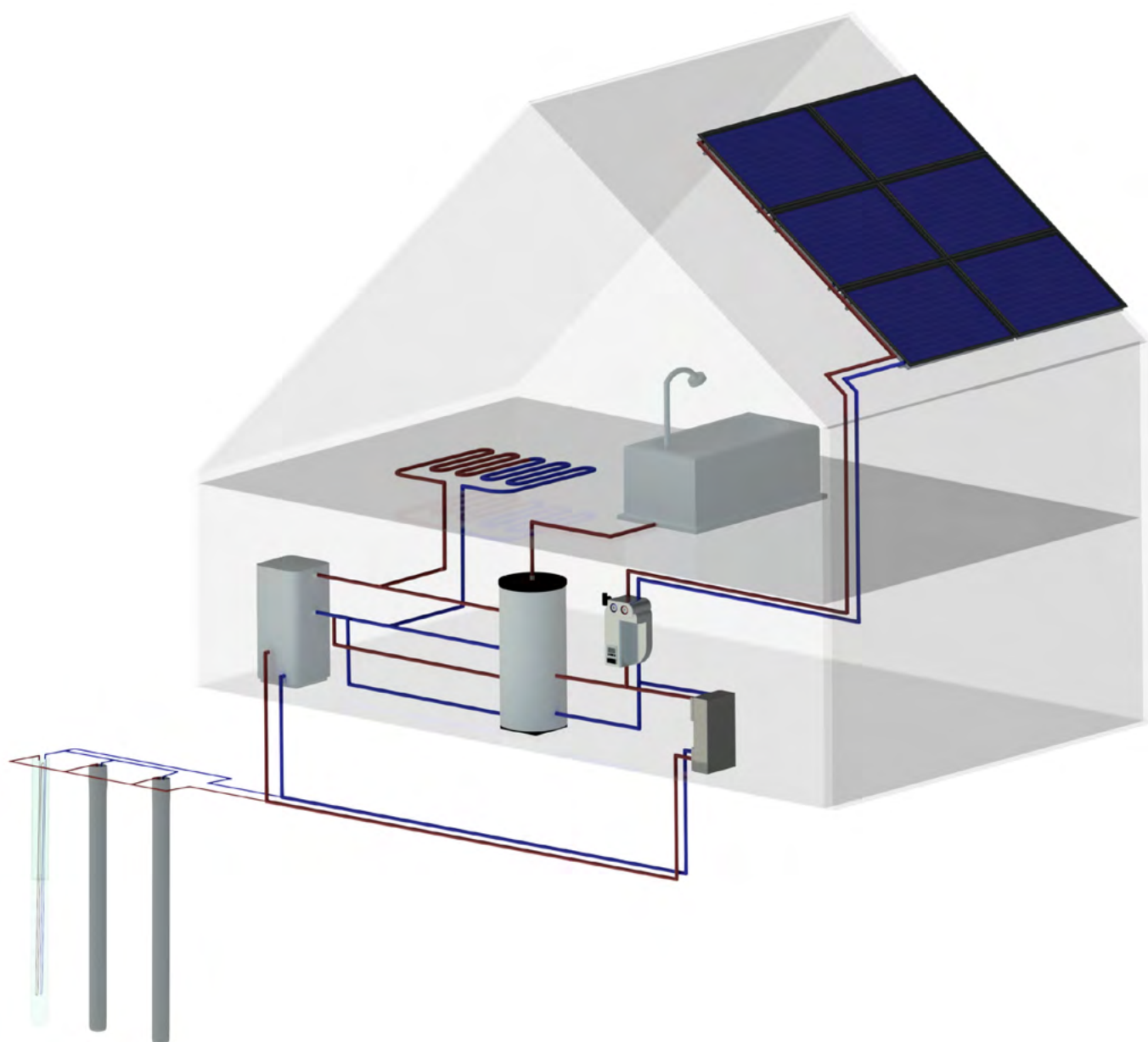
Schéma de l'installation
